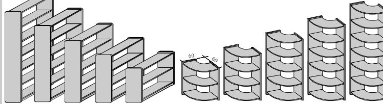
R-7 R-6 R-5 R-4 R-3 RR-3 RR-4 RR-5 RR-6 RR-7 210-90-30 175-90-30 145-90-30 110-90-30 76-90-30 výška 76 110 145 175 210
